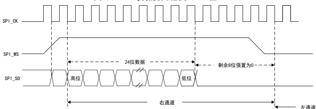
图 99 I2S 飞利浦协议波形（24 位）
