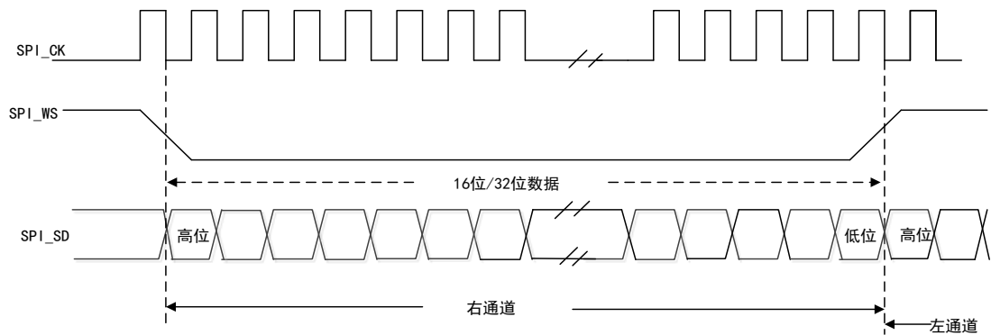
图 101 MSB 对齐标准波形（16/32 位数据）
