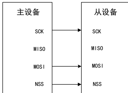
图 96 单工模式连接（主机只发送，从机接收）
