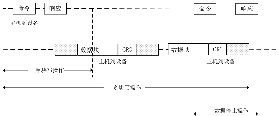
图 121 SDIO (多) 数据块写操作
