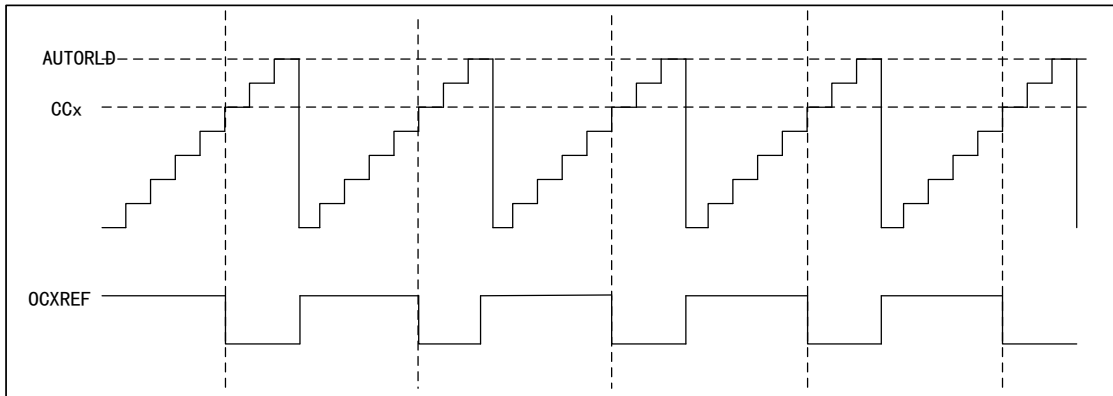
图 48 PWM1 向上计数模式的时序图
