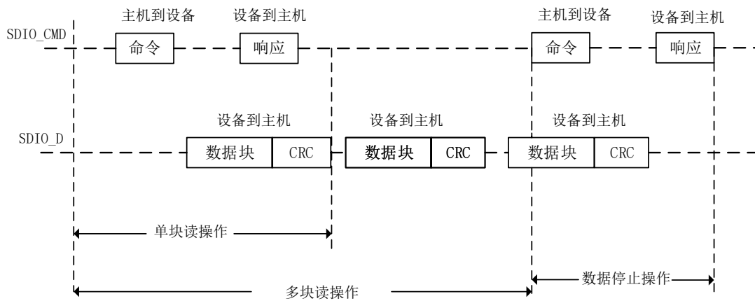
图 120 SDIO (多) 数据块读操作
