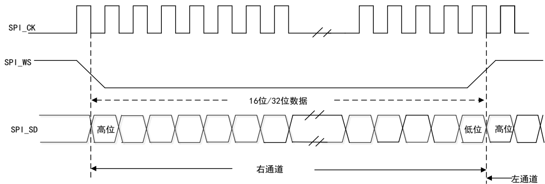
图 104 LSB 对齐标准波形（16/32 位数据）
