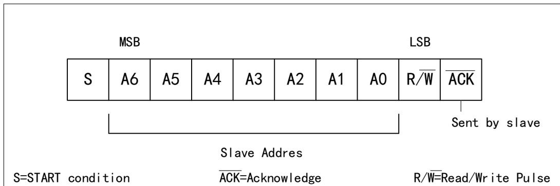
图 86 7 位地址格式
