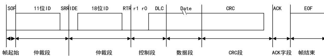
图 110 扩展数据帧
