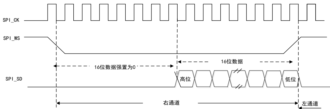
图 106 LSB 对齐标准下（16 位扩展至 32 位）
