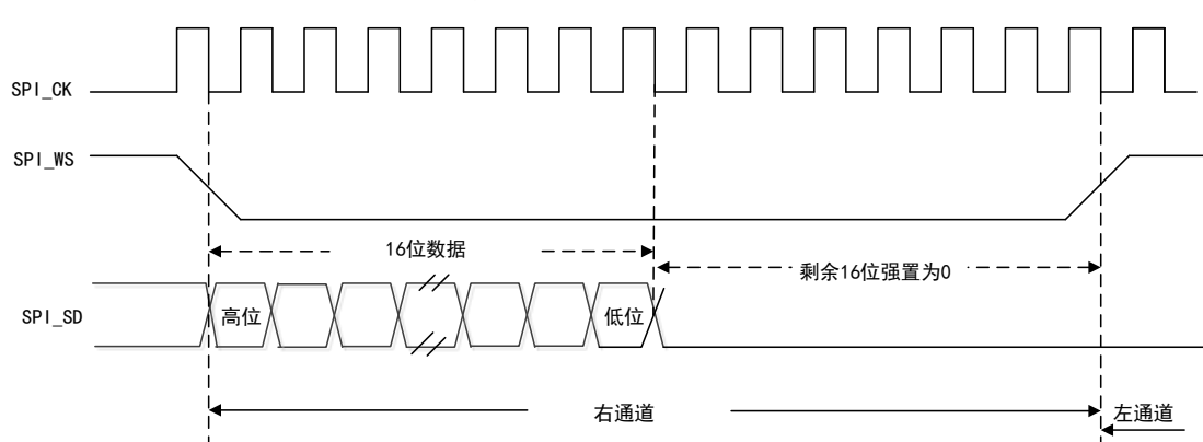
图 103 MSB 对齐标准波形（16 位扩展至 32 位）
