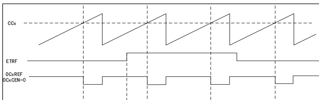
图 42 OCxREF 时序图
