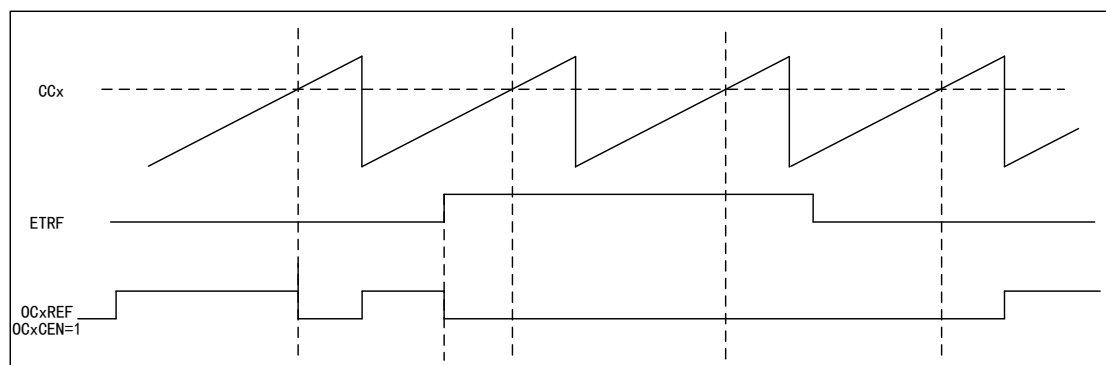
图 59 OCxREF 时序图
