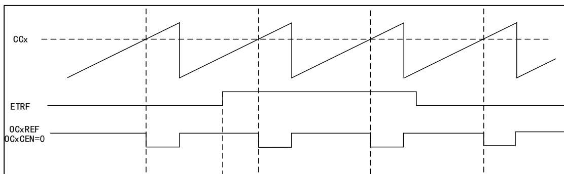
图 58 OCxREF 时序图
