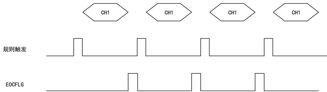
图 126 单次转换模式时序图
