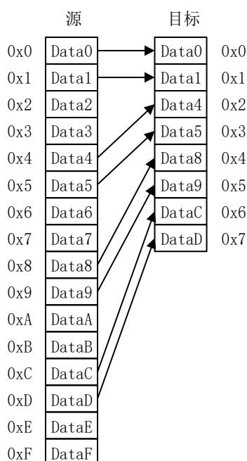
图 16 源为 32bits 目标为 16bits 的传输宽度
